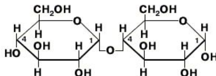
Мальтоза
