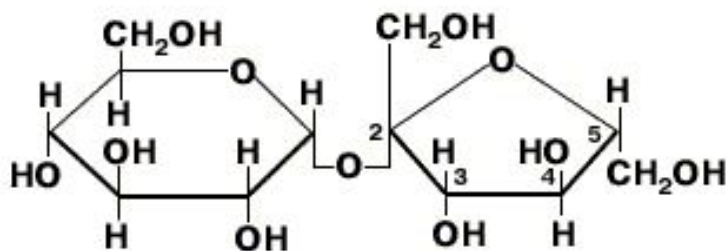
Сахароза
