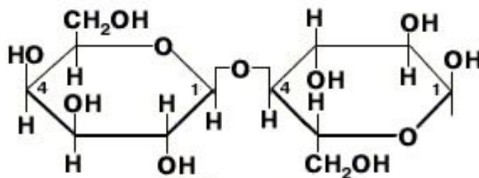
Лактоза
