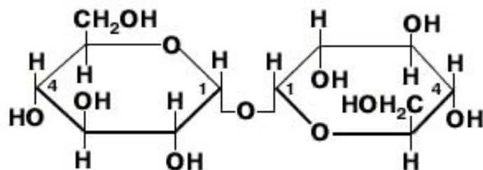
Трегалоза
