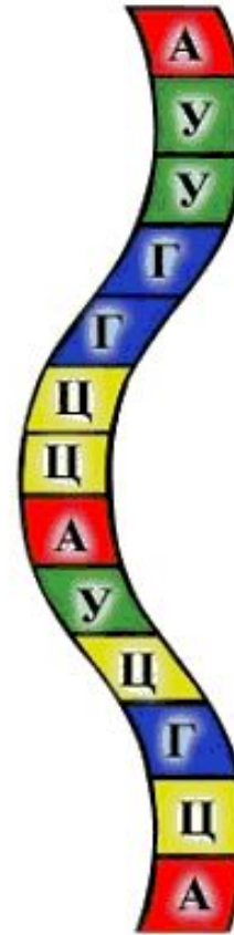
РНК
