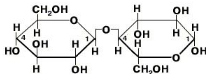
Целлобиоза
