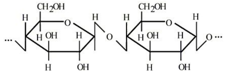
Структурная формула ЦЕЛЛЮЛОЗЫ
