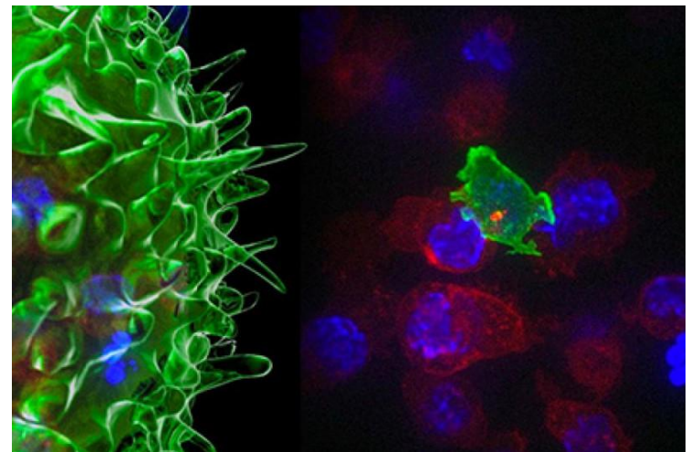
Т-хелперы
