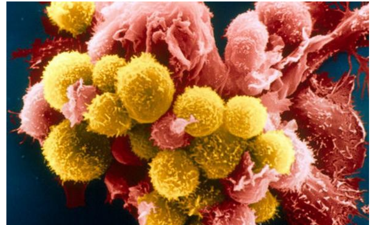
Т-хелперы
