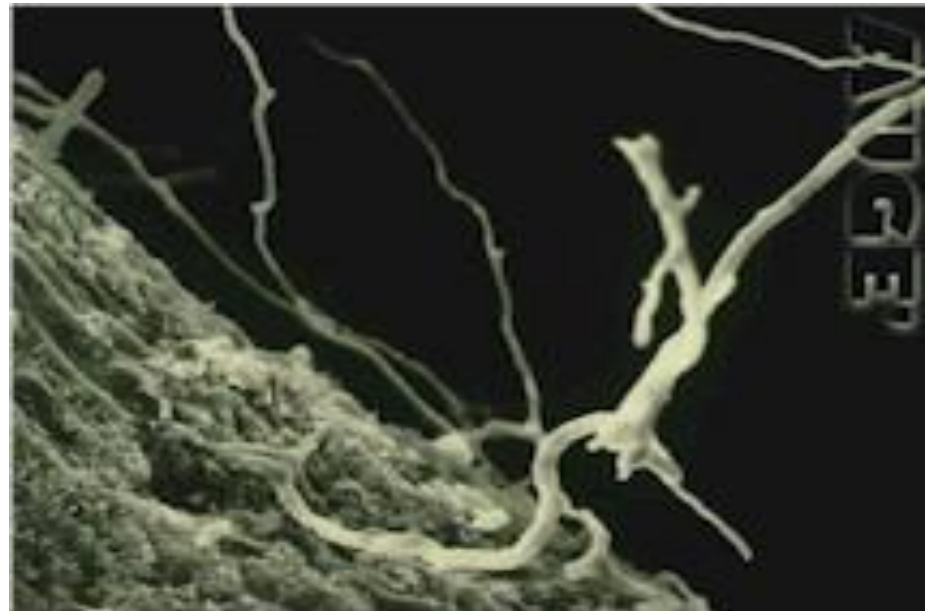
Glomus deserticola
