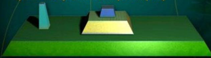
Пирамида продукции луга – единица измерения кДж/м^2/год
