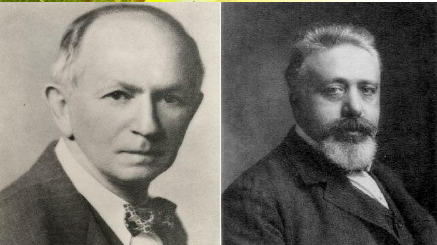
МОДЕЛЬ ЛОТКИ-ВОЛЬТЕРРА (по К. Вилли)
