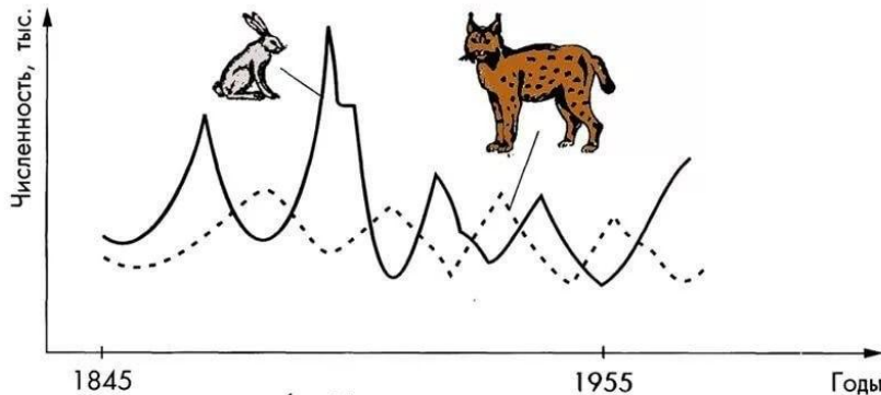
МОДЕЛЬ ЛОТКИ-ВОЛЬТЕРРА (по К. Вилли)
