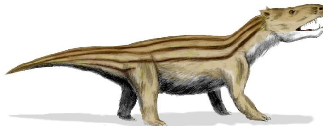
цинодон
