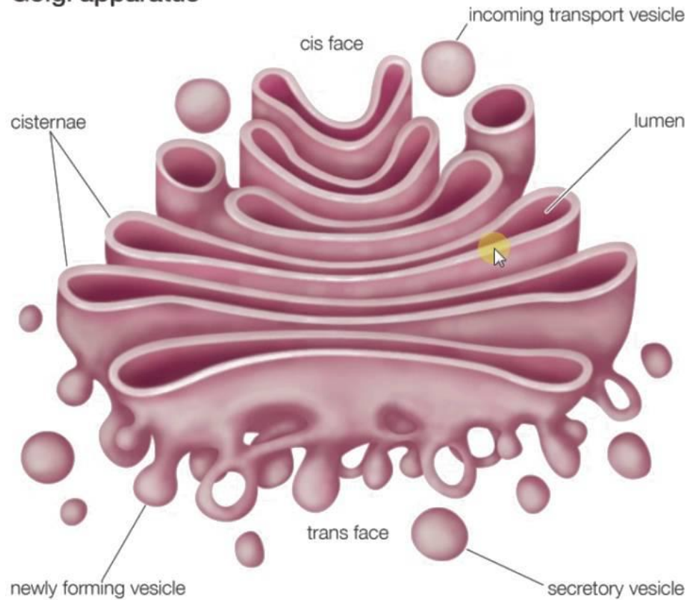
Golgi apparatus
