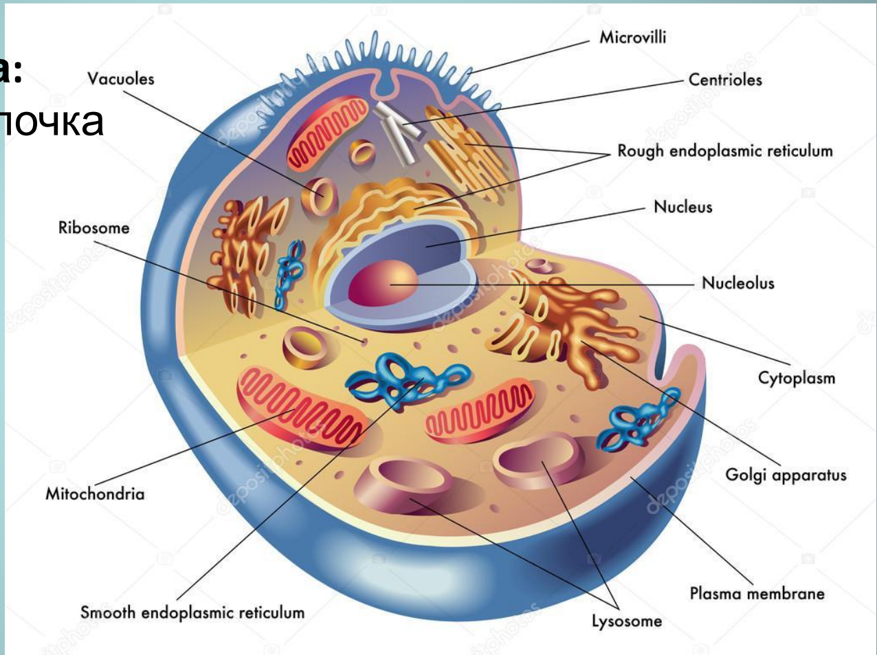
Рис. 1 Строение клетки
