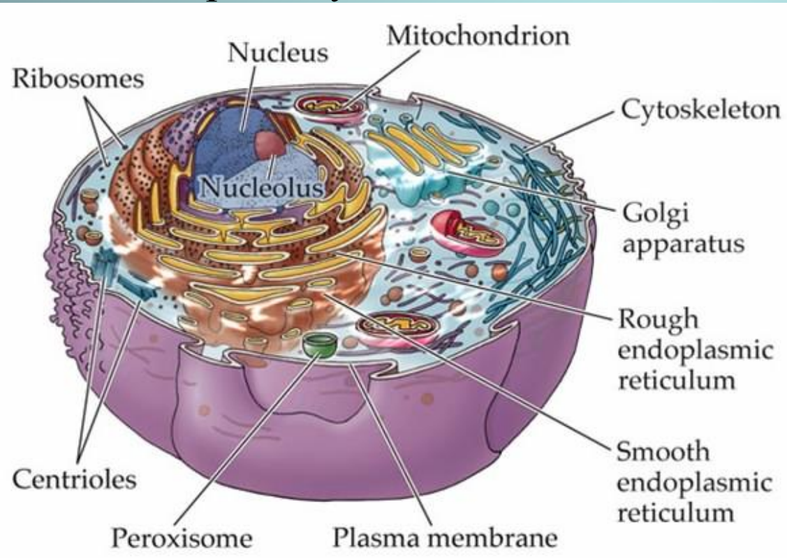
Рис. 4 Строение ЭПС
