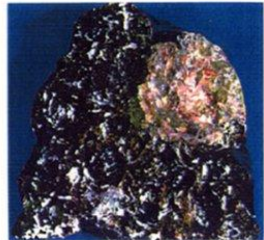
Ткань легкого курящего человека
