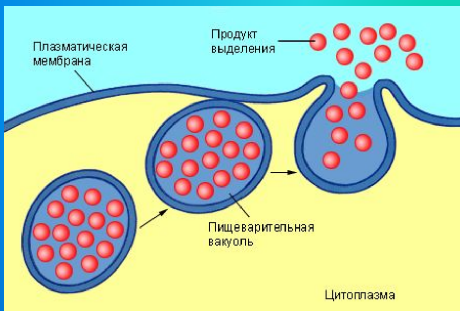
Экзоцитоз
