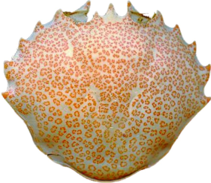
Карапакс краба
