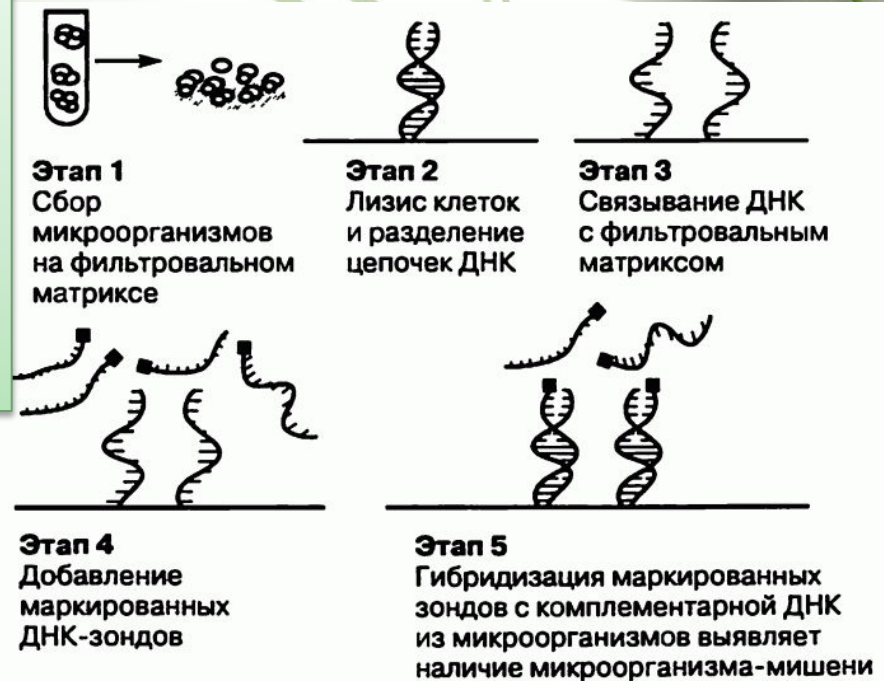
Рис. 8.4. Тест ДНК–ДНК-гибридизации
