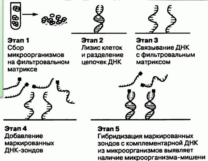
Рис. 8.4. Тест ДНК–ДНК-гибридизации
