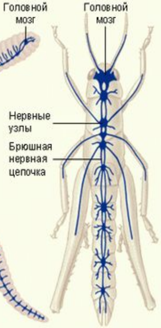
Насекомое
