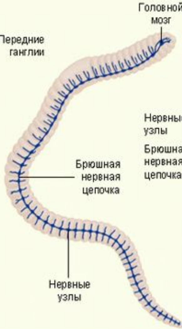
Дождевой червь
