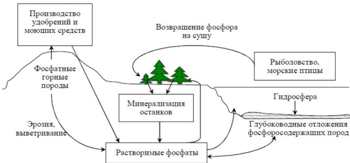
Круговорот фосфора и серы
