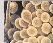
споры грибов
