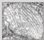
митохондрия x900000
