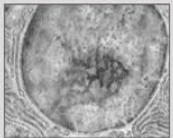
ядро x20000
