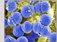
стрептококк
