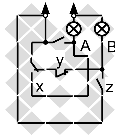
Электрическая схема
