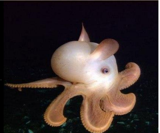
Осьминог думбо
