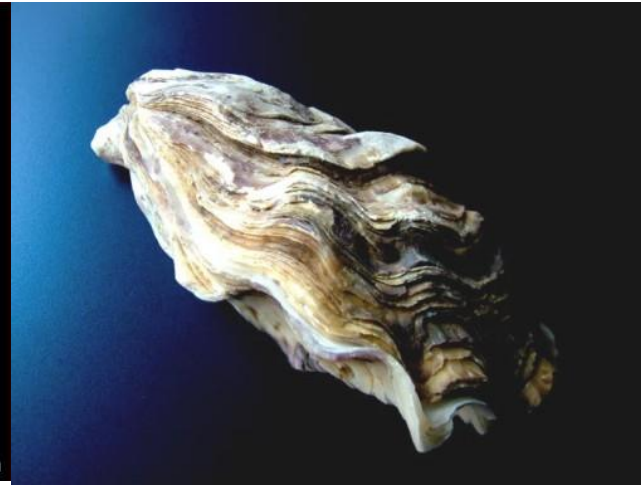
Устрица
