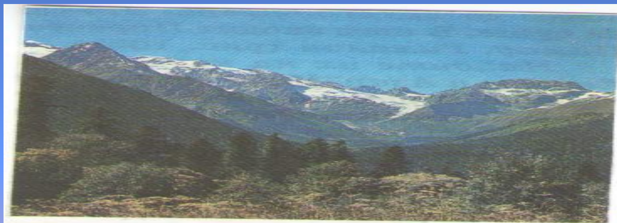
Рис. 105. Кавказские горы — часть Альпийско-Гималайского складчатого пояса
