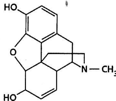
Морфин
