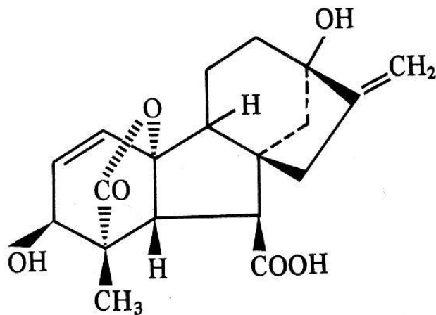
гиббереллин
