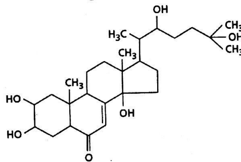
\alpha -Экдизон
