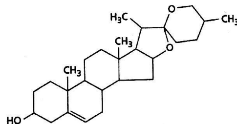
Ямогенин
