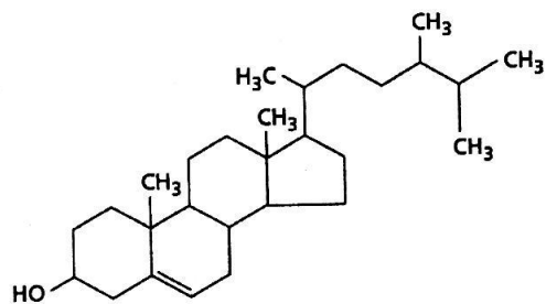
Ситостерол
