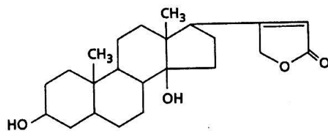
Дигитоксигенин
