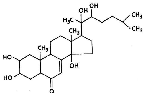
Понастерон А
