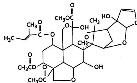
Азадирахтин
