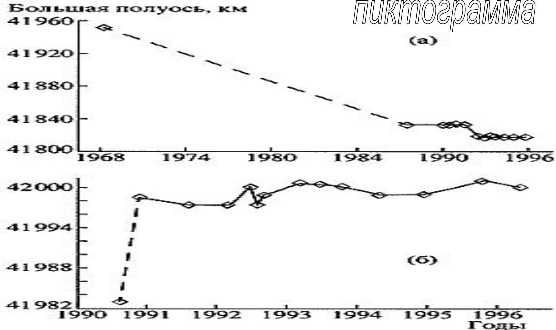
Изменение большой полуоси орбиты геостационарных искусственных спутников Земли "Транс-тэйдж-13" (а) и "Горизонт-21" (б)
