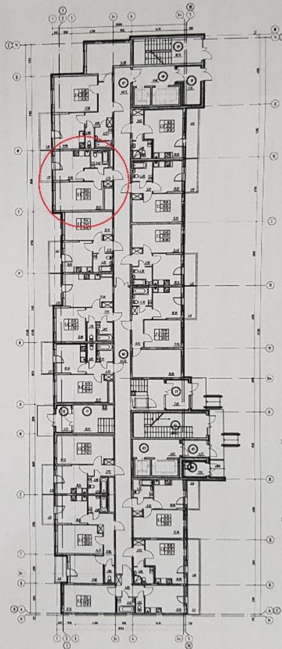
Корпус 2. Секция 3 План 1-го этажа
