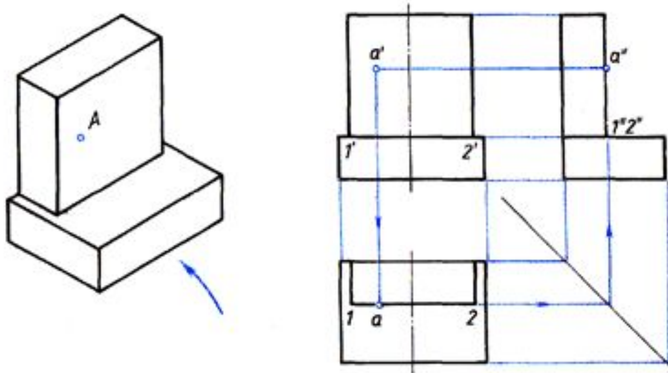
Рис. 156. Построение проекций точки, заданной на поверхности детали
