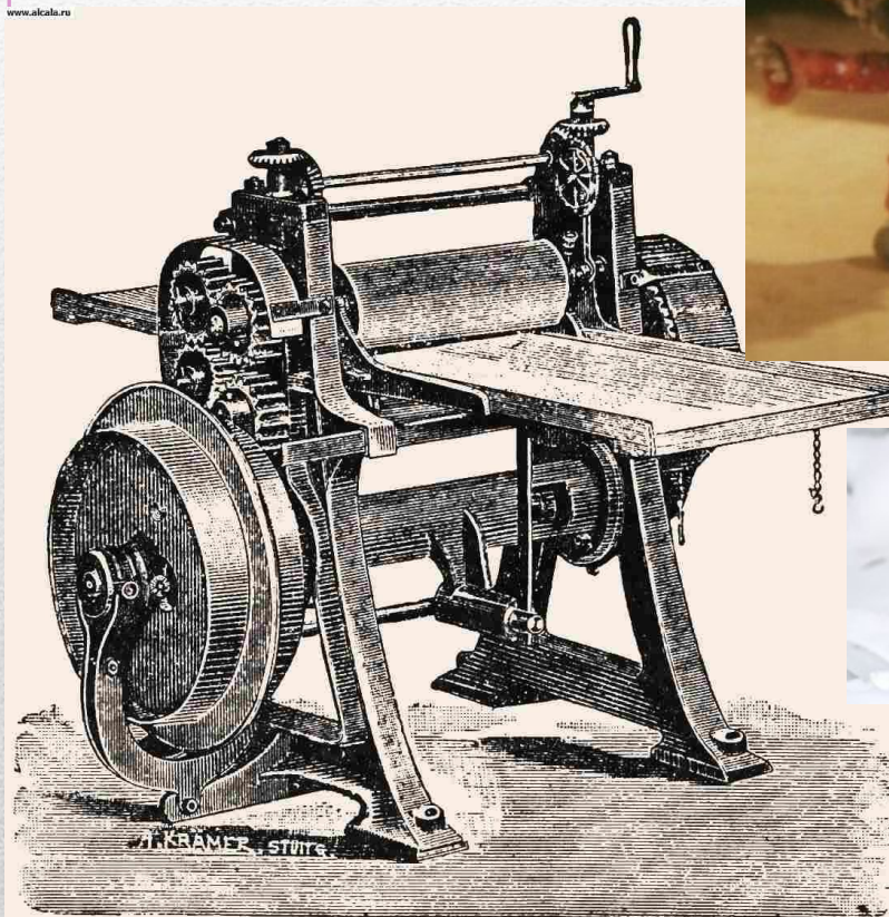
Фиг. 3. Вальцы со столикомъ для прокатки листовъ.
