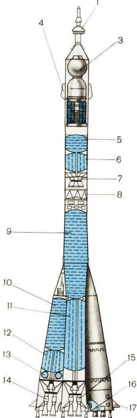
Ракета-носитель «Союз»
