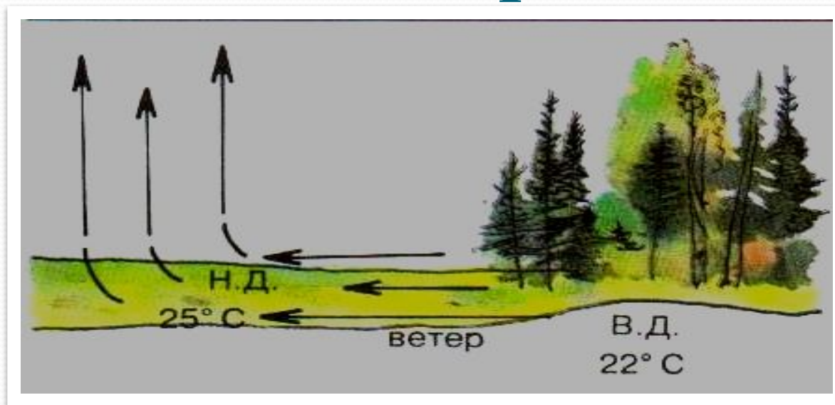
Образование ветра в жаркий летний день
