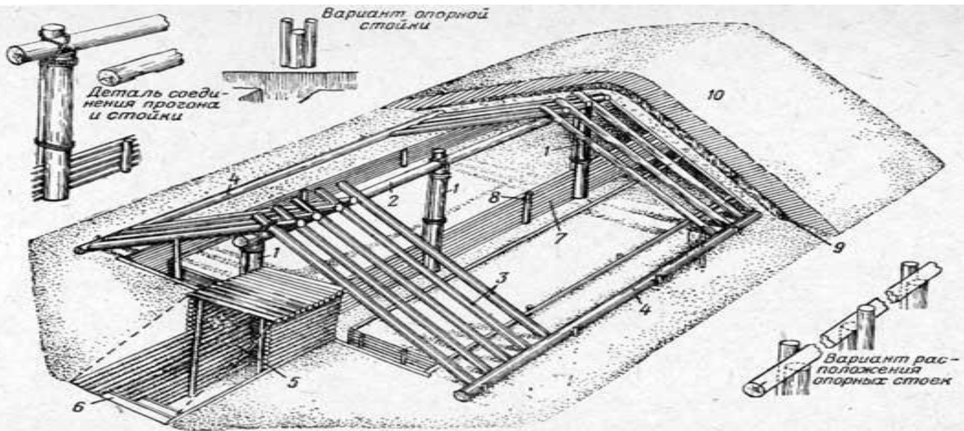
Рис. 19. Устройство двускатной землянки:
