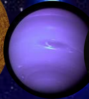
Нептун
