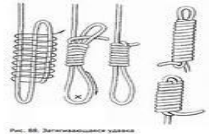
Рис. 88. Затягивающиеся узлы
