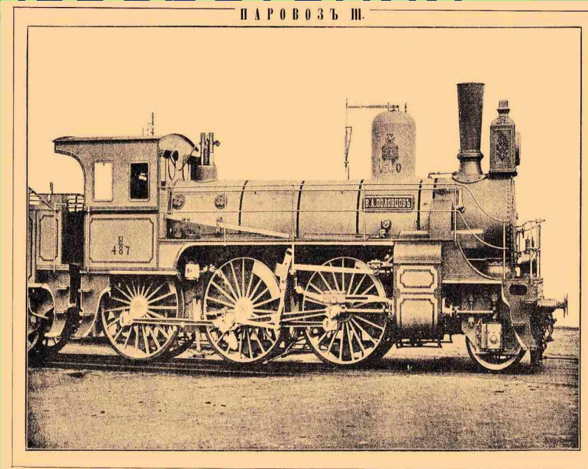
Четырехосный паровоз кокаунд, с одной поддерживающей осью, серия И Николаевской ж.д. д.р.
