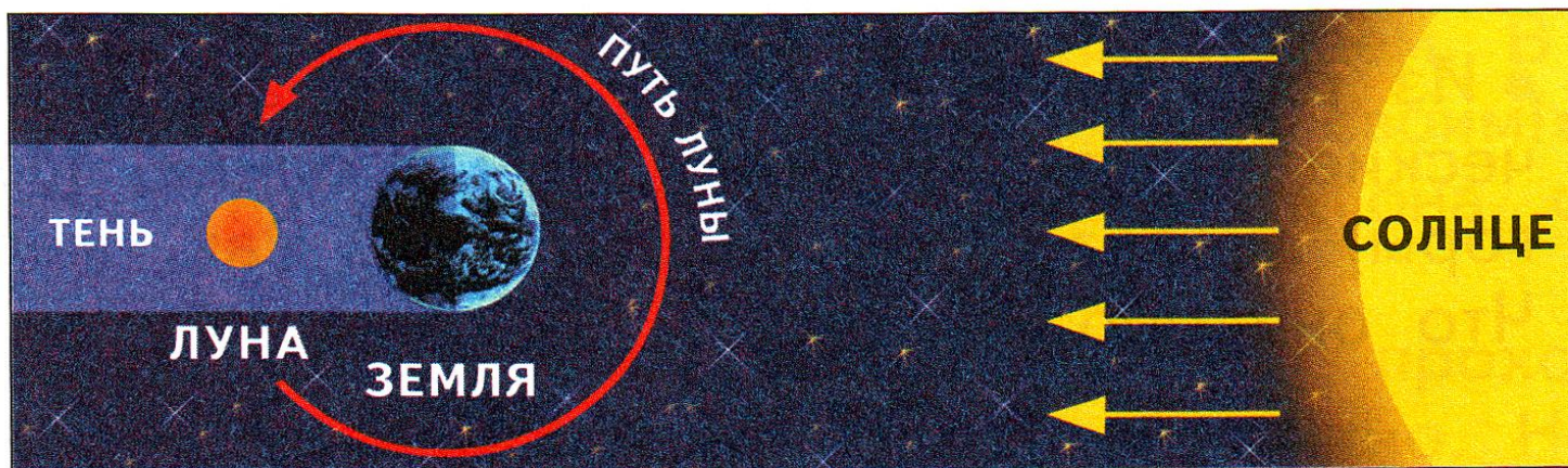
▲ Схема лунного затмения
