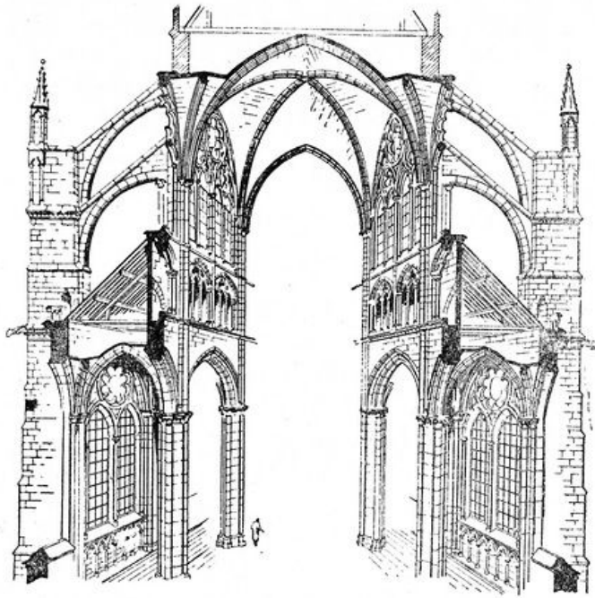
Поперечный разрез готического собора
