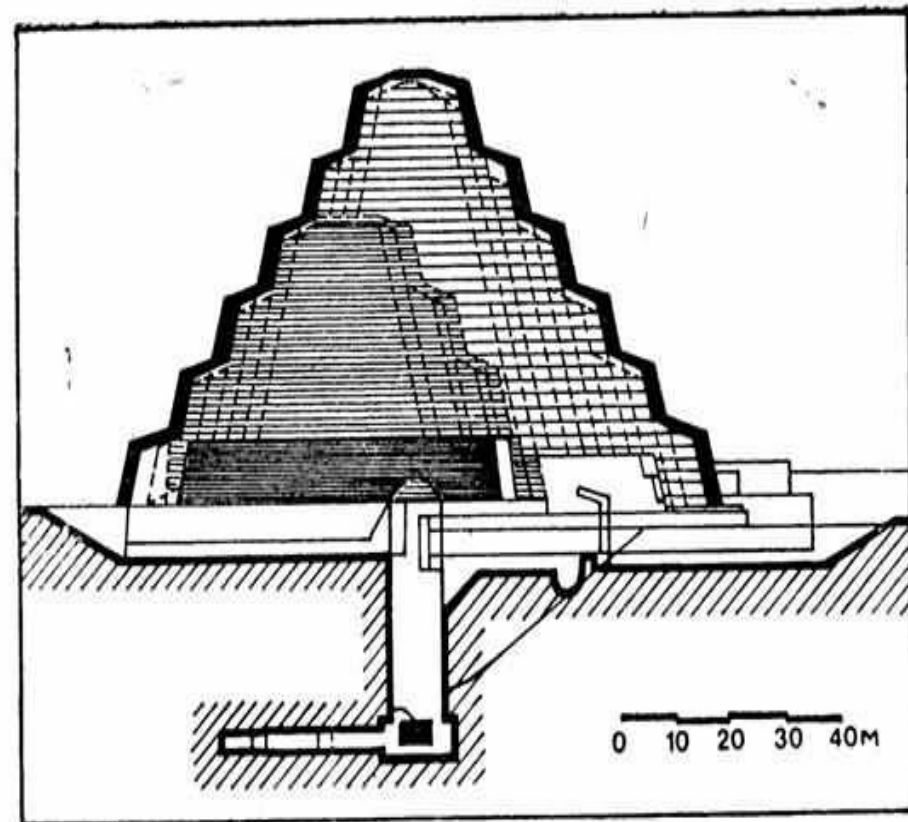
Пирамида Джосера в Саккара. Разрез, иллюстрирующий отдельные стадии строительства (по Лауэру)
