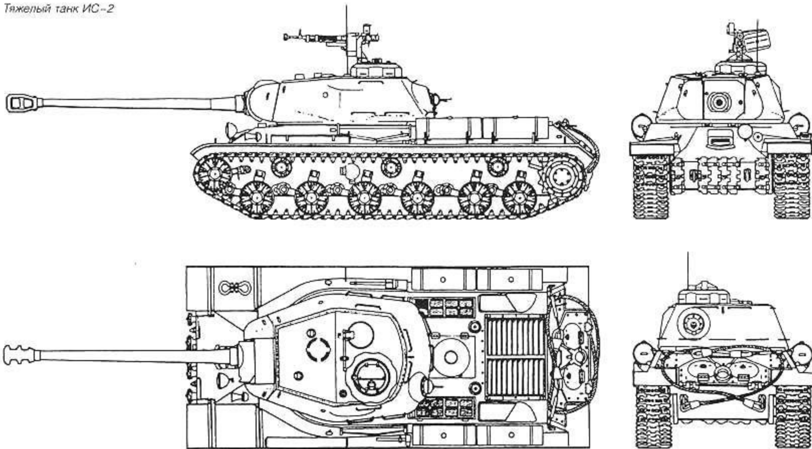
Тяжелый танк ИС-2
