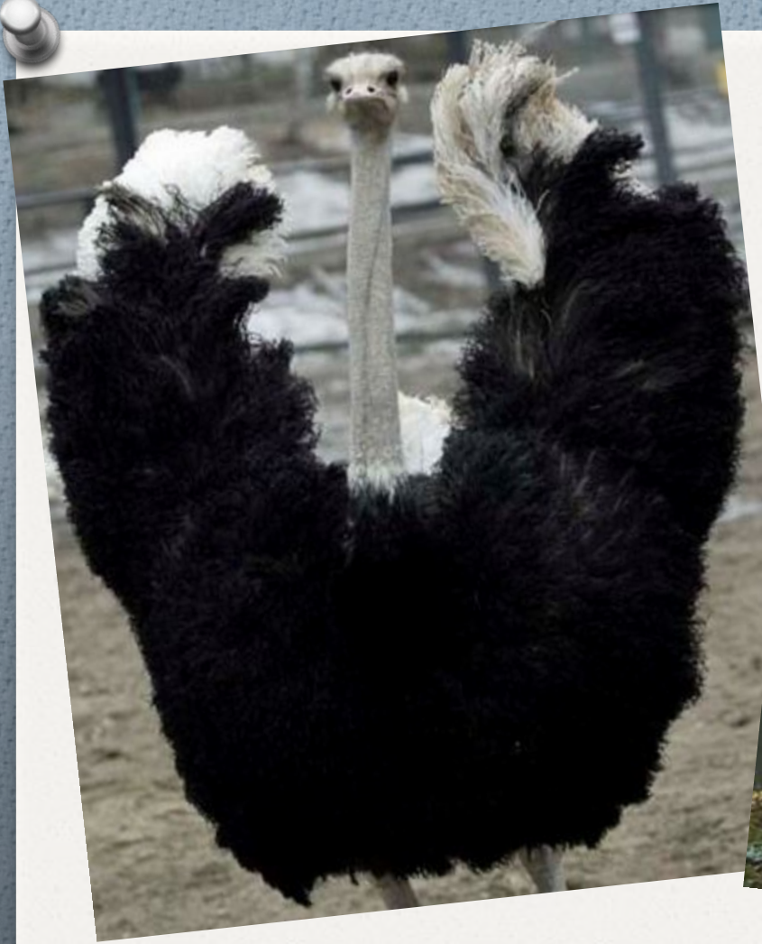
страус
