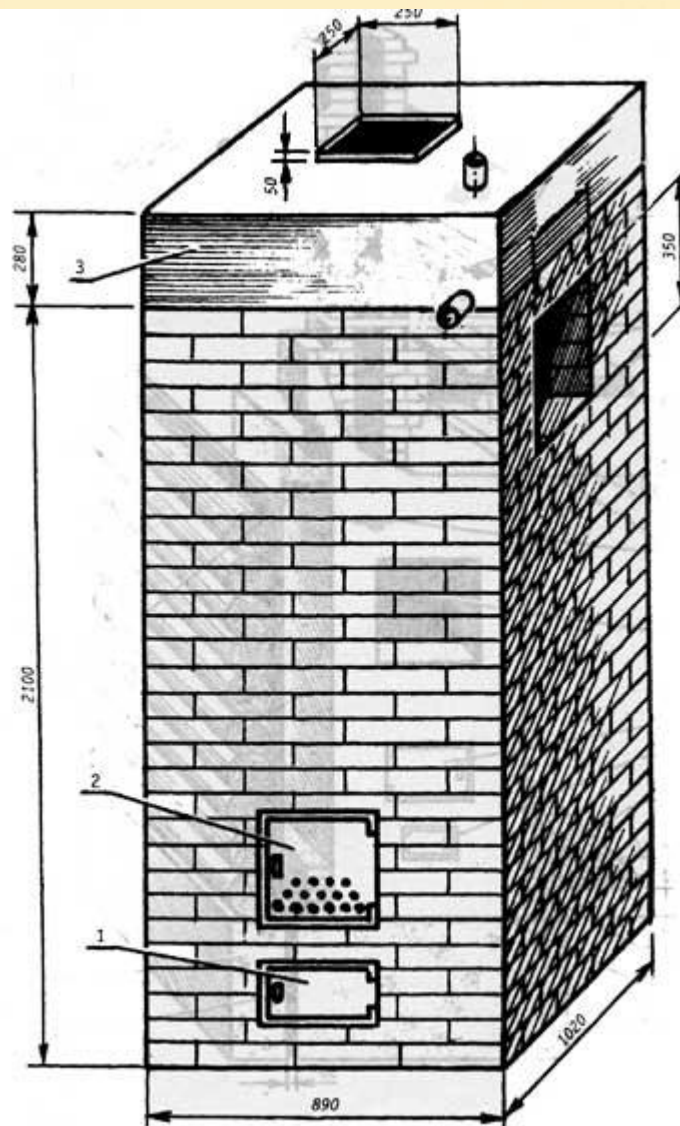
Рис. 5.2.2. Внешний вид печи-каменки: 1 – поддувало; 2 – топливник; 3 – бак для воды
