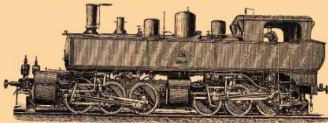
3. Двойной танковый паровоз, системы компаунда, Сент-Готтардской жел. дор.
