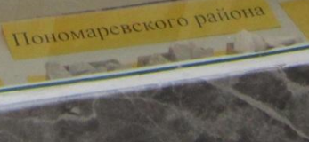
Полезные ископаемые
