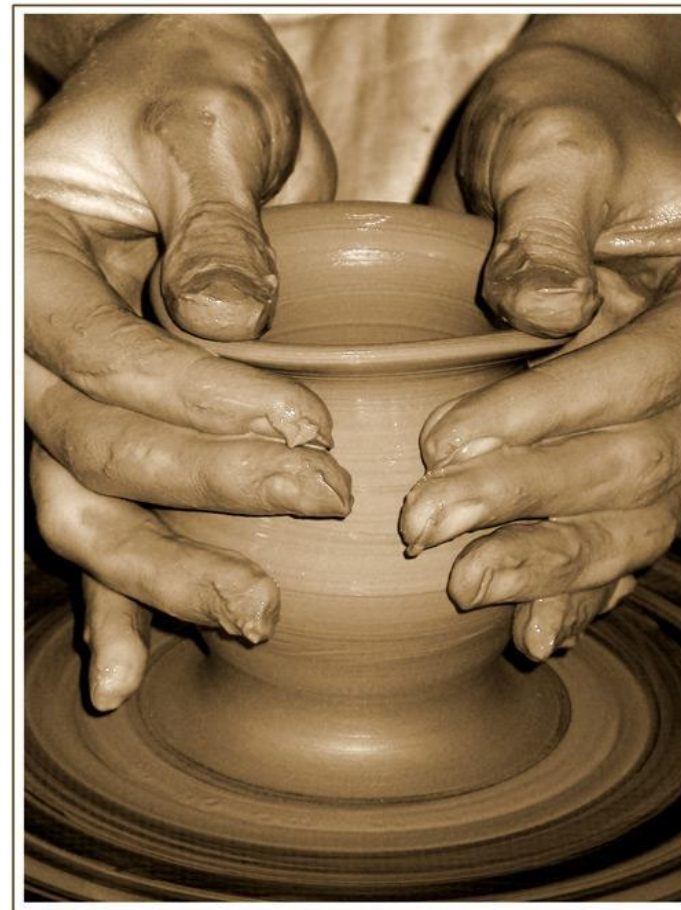
Ремесло гончара.
