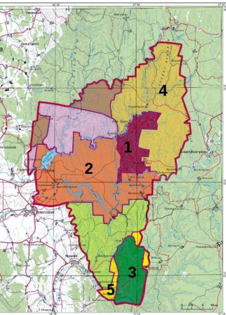
КАРТА 2. СТРУКТУРА БИОСФЕРНОГО РЕЗЕРВАТА «БАШКИРСКИЙ УРАЛ»
