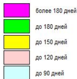
Рис. 5. Территориальные различия количества инверсий в году в Кемеровской области
