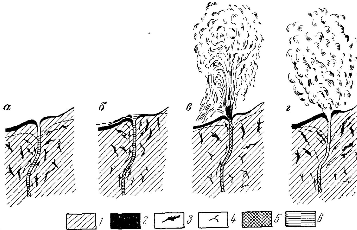
Рис. 116. Основные стадии действия камчатских гейзеров (по Т. И. Устиновой): 1 — непловые туфы; 2 — отложения гейзерита; трещины в туфах: 3 — с перегретой водой, 4 — с охлажденной водой; 5 — перегретая вода с температурой выше 100° С; 6 — охла- жденная вода с температурой ниже 100° С
