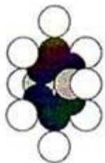
Ядро атома кислорода
