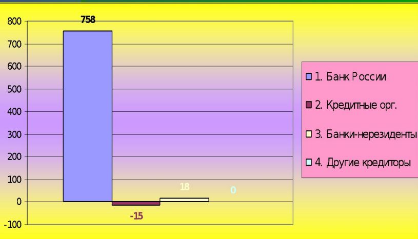
Рис. 14. Динамика темпа прироста процентных расходов банка за 2008-2009 гг., %
