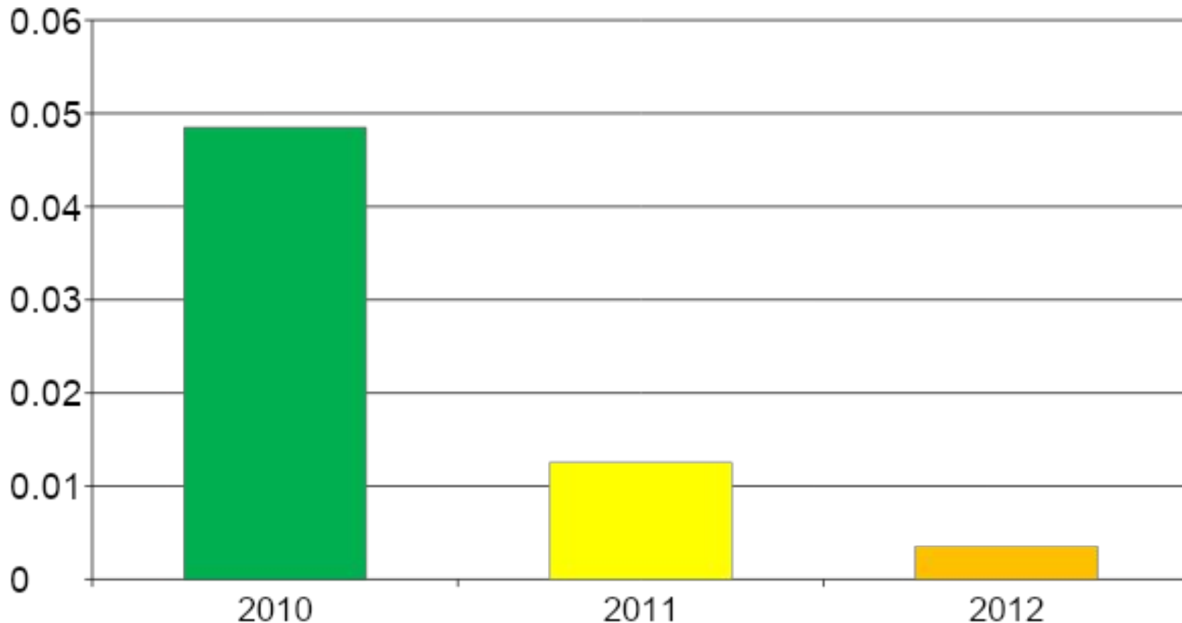
Рентабельность активов
