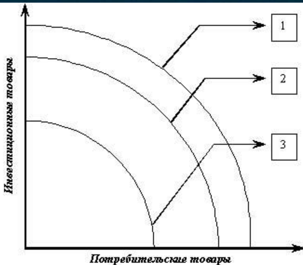
Рис. 1. Кривые возможностей
