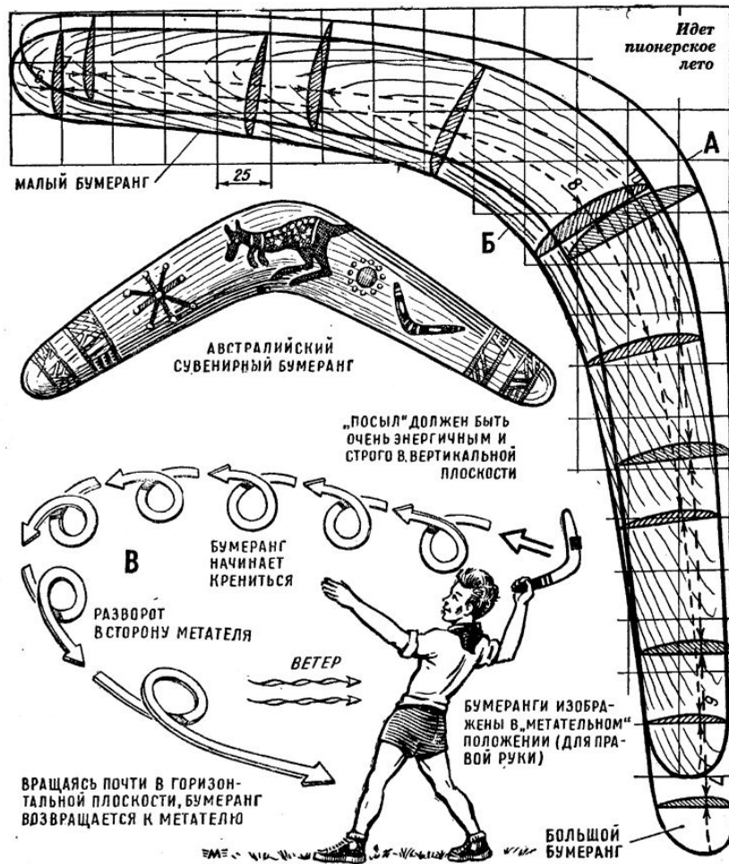
Рис. 2. Контуры спортивно-олимпийских бумерангов, спроектированных чемпионом Австралии Джо Тимберли: А — для взрослых спортсменов, Б — для детей и женщин, В — схема выполнения броска «нормальная петля».
