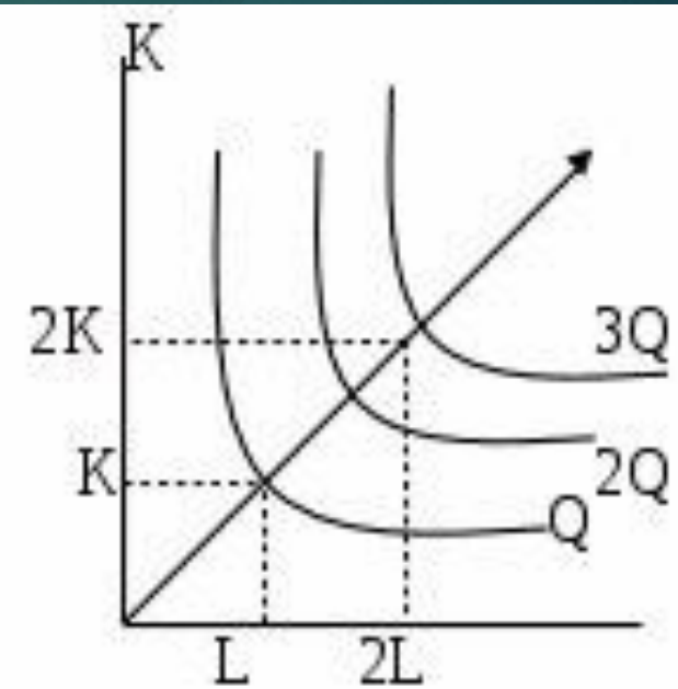
Убывающая отдача
