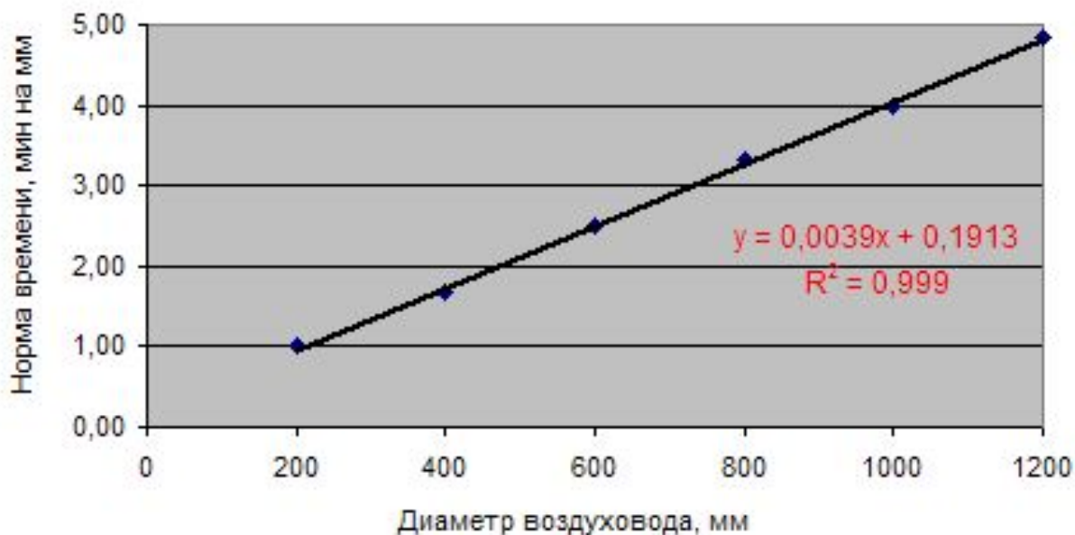
График зависимости нормы времени изготовления спирально-навивных воздуховодов от диаметра трубы
