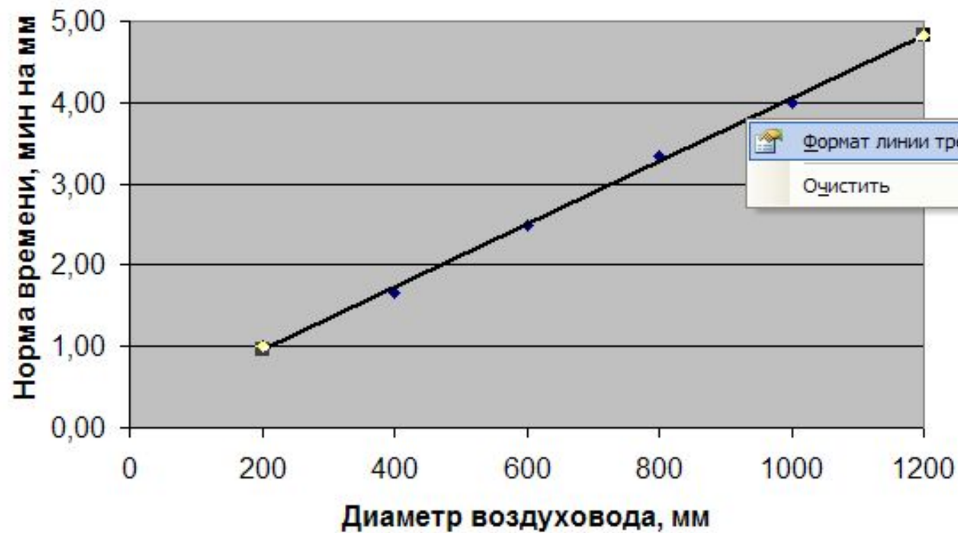
График зависимости нормы времени изготовления спирально-навивных воздуховодов от диаметра трубы
