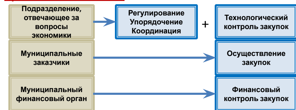
Предлагаемая модель 3.
