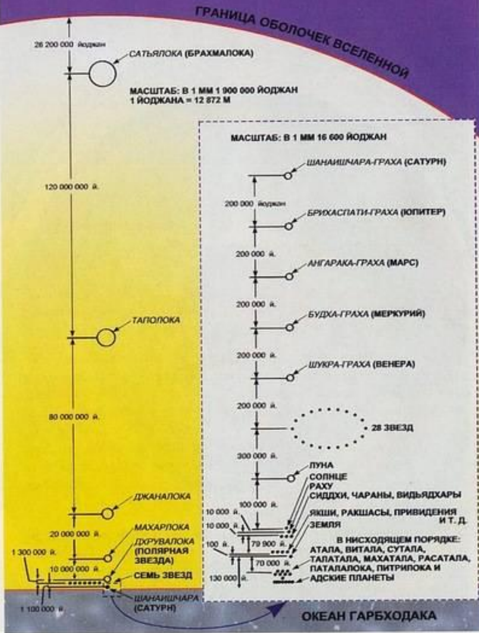
Схема расположения различных планет вселенной.
