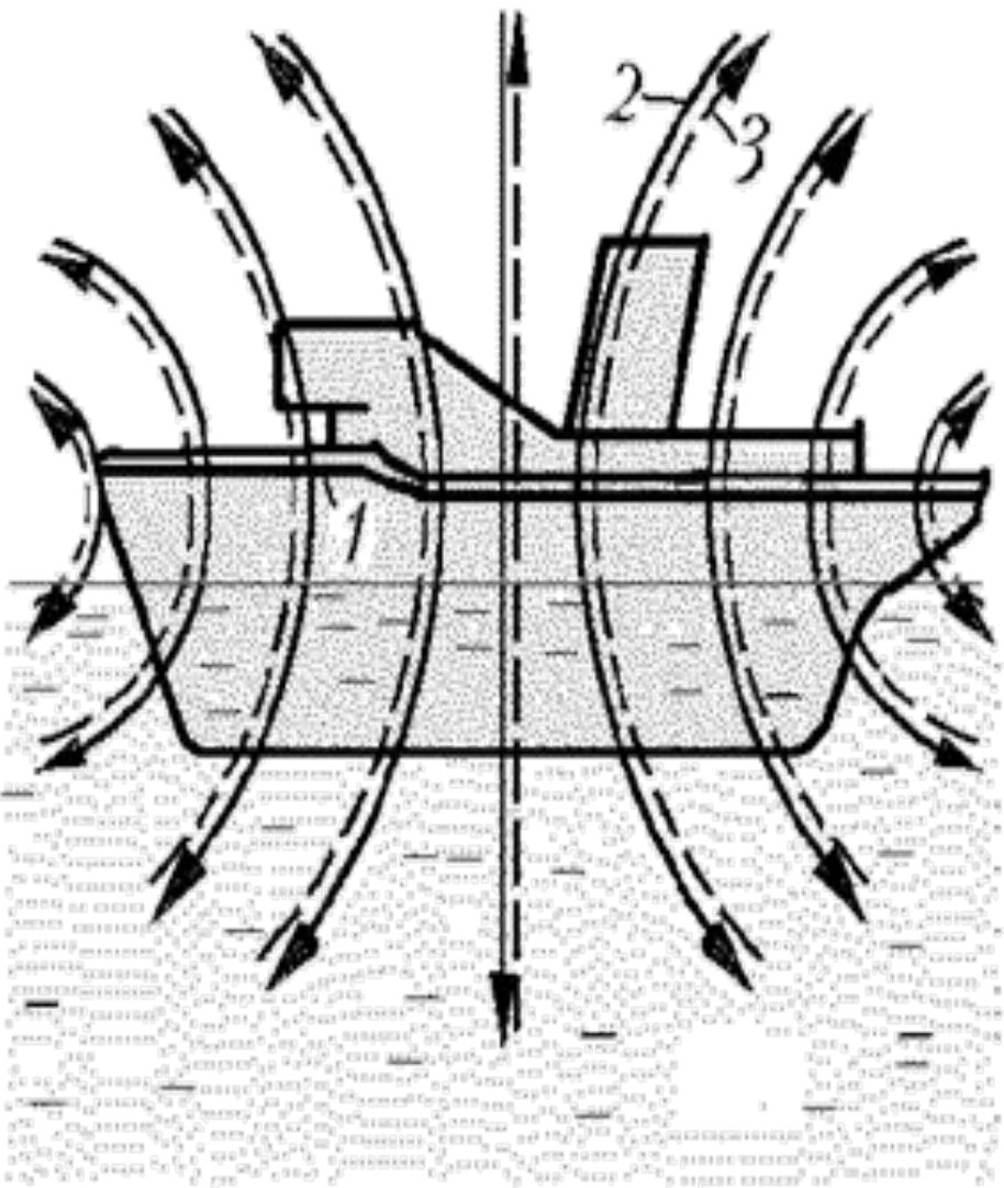
Обмоточный метод размагничивания судов
